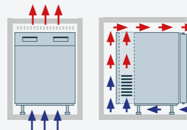
D: Lufteinlass unter und Auslass direkt über der Minibar
