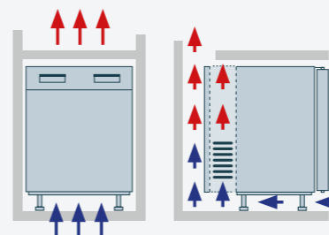
C: Lufteinlass unter der Minibar und Auslass über Lüftungsschlitz oberhalb
