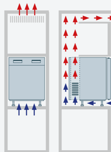
A: Lufteinlass unter der Minibar und Auslass über ein darüber gelegenes Fach
