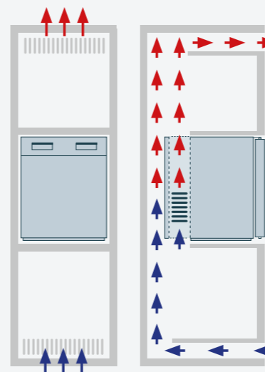
B: Lufteinlass unter und Auslass über einem Fach, freie Zirkulation entlang der gesamten Rückwand
